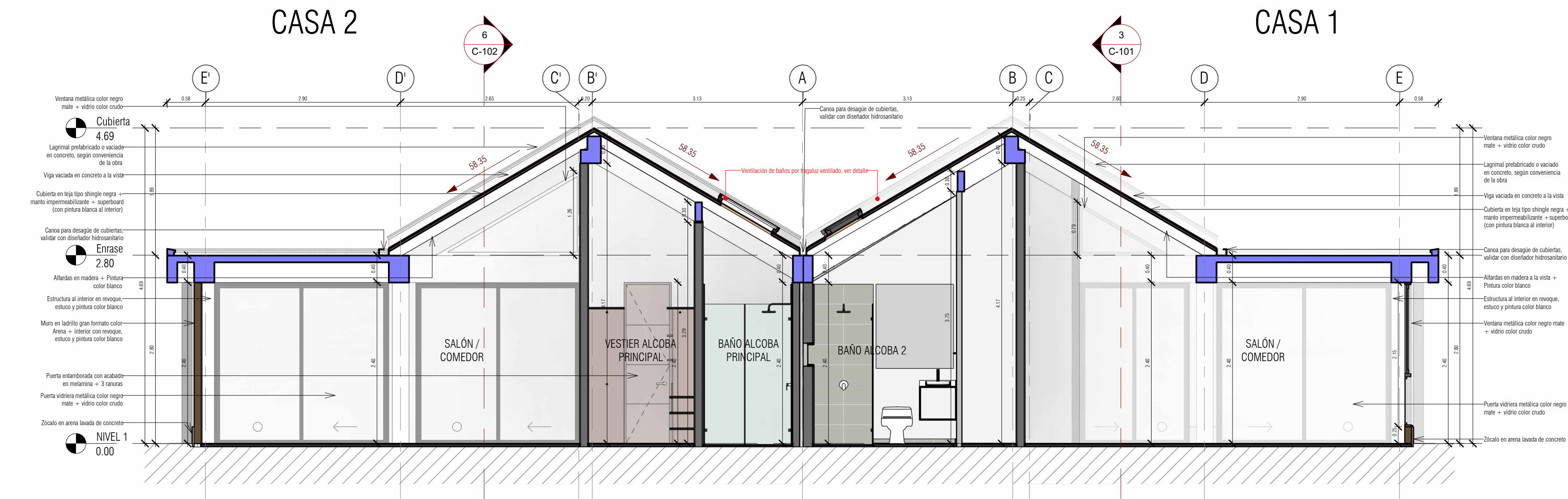
2 SECCIÓN TRANSVERSAL - CASAS 1 Y 2 1:50
