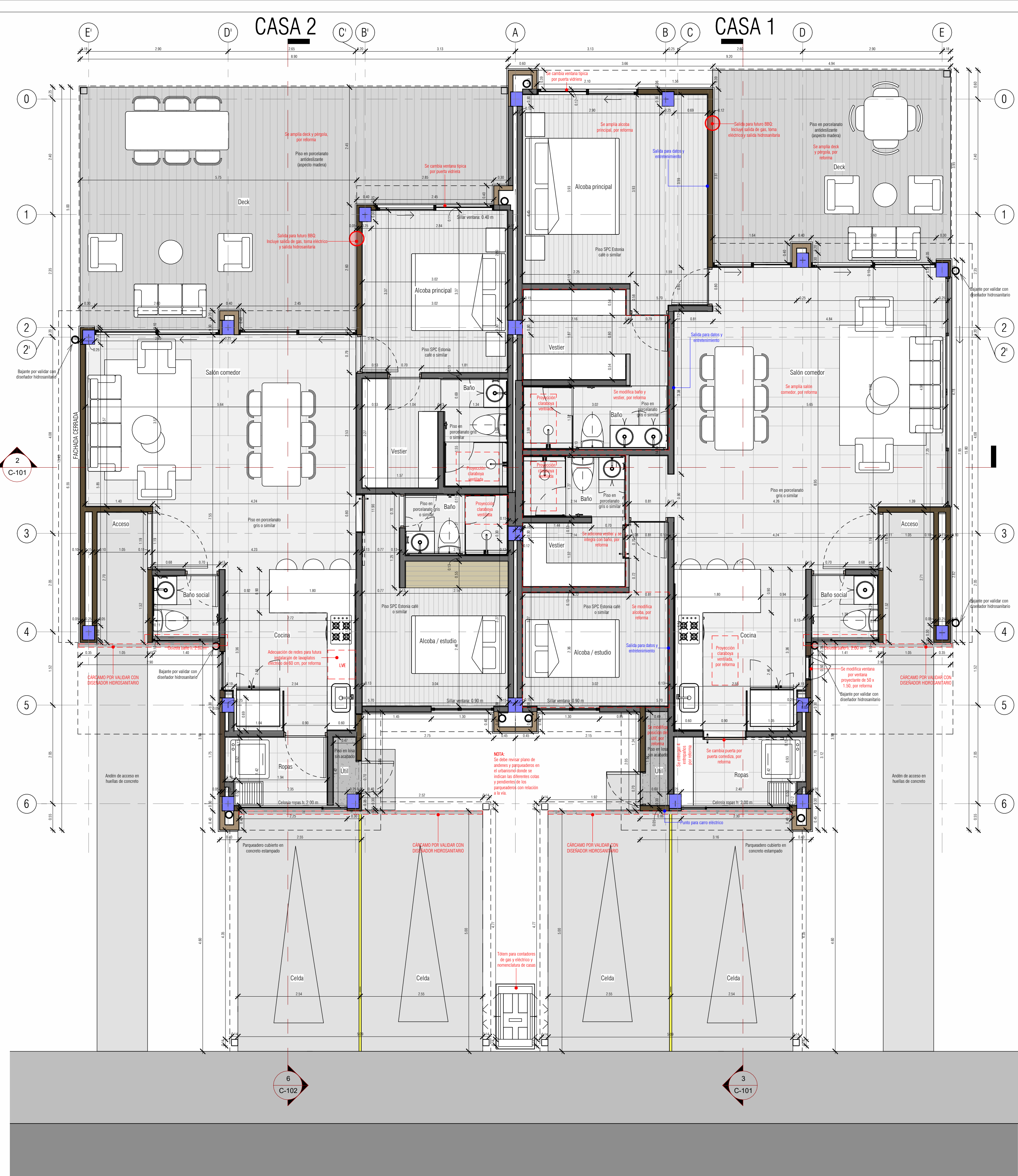
1 PLANTA - CASAS 1 Y 2 1:50
