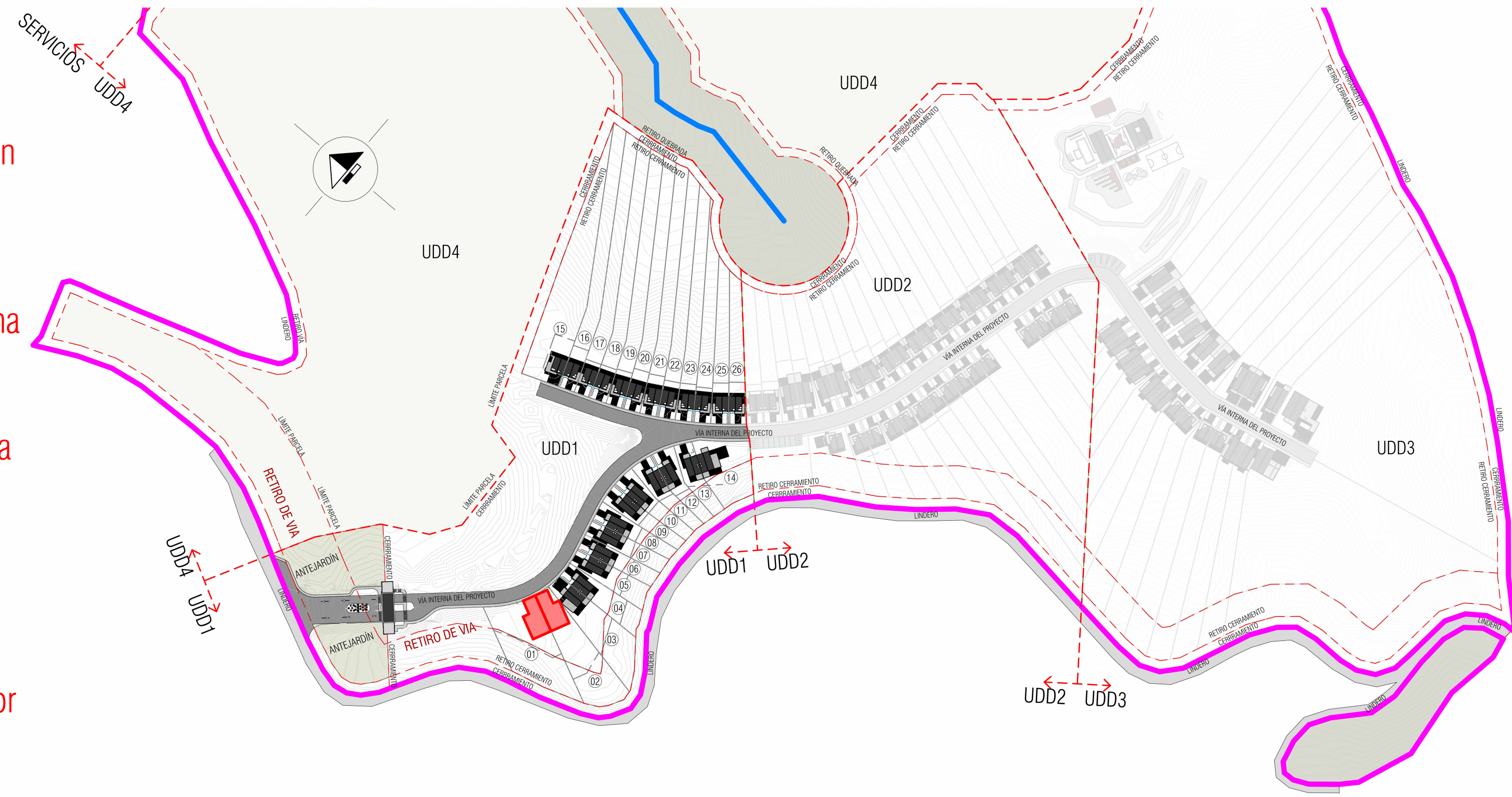
LOCALIZACIÓN CASAS 1 Y 2 1:1
